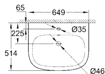
39 323 000 39 323 00H* Lavabo suspendu 65 cm
