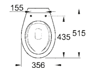
39 430 000 WC posé au sol sans rebord
