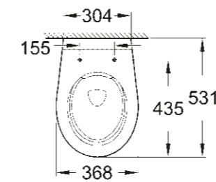
39 427 000 WC suspendu sans rebord
