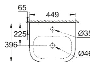
39 324 000 39 324 00H* Lave-main 45 cm
