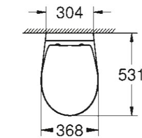
39 351 000 WC suspendu sans rebord Siège et abattant avec frein de chute Fonction déclinable
