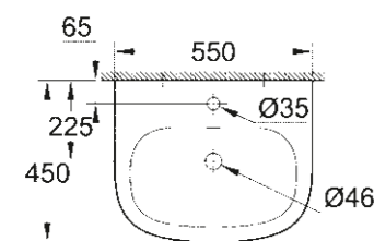
39 336 000 39 336 00H* Lavabo suspendu 55 cm
