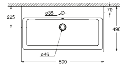
39 478 00H Vasque à poser 50 cm
