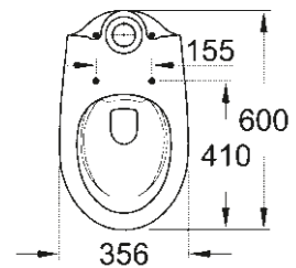
39 349 000 WC posé au sol pour combinaison monobloc sans rebord, sortie horizontale
