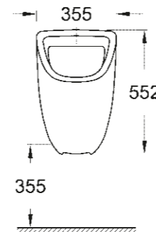
39 439 000 Urinoir avec alimentation apparente par le haut
