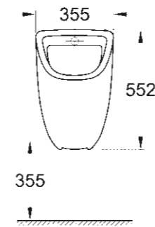
39 438 000 Urinoir avec alimentation encastrée
