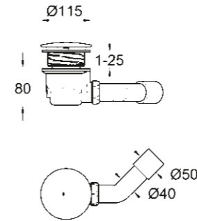
49 534 000* Clapet de vidage horizontal pour bacs de douche universels
