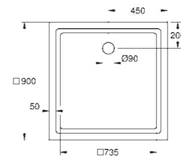
39 301 000* Bac de douche universel 90 cm x 90 cm
