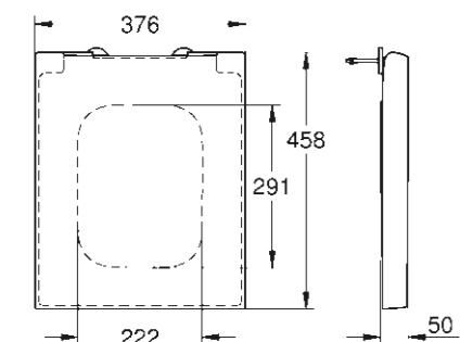
39 488 000 Siège et abattant avec frein de chute Fonction déclipable
