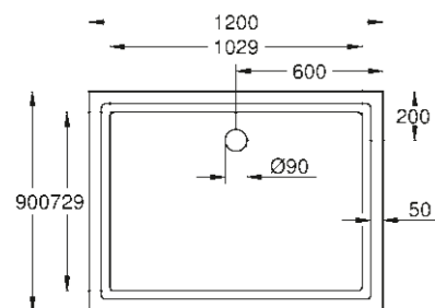
39 308 000* Bac de douche universel 90 cm x 120 cm
