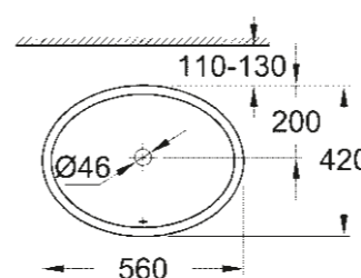
39 423 000 Vasque à encastrer par le dessus 55 cm
