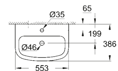
39 440 000 Lavabo suspendu 55 cm
