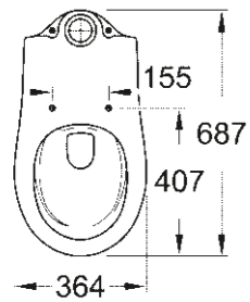
39 429 000 WC posé au sol pour combinaison monobloc sans rebord, sortie verticale
