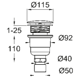
49 533 000* Clapet de vidage vertical pour bacs de douche universels
