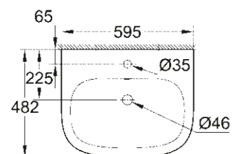
39 335 000 39 335 00H* Lavabo suspendu 60 cm
