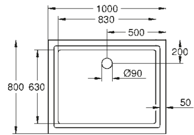
39 306 000* Bac de douche universel 80 cm x 100 cm
