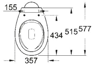
39 431 000 WC posé au sol sans rebord
