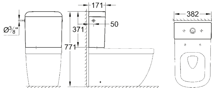
39 333 000 Réservoir de chasse avec entrée latérale et arrière
