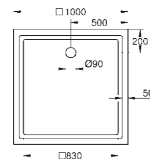
39 300 000* Bac de douche universel 100 cm x 100 cm
