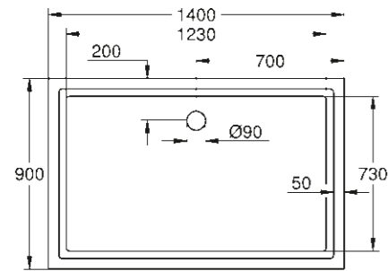
39 307 000* Bac de douche universel 90 cm x 140 cm
