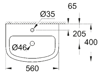
39 422 000 Lavabo à encastrer par le dessus 55 cm
