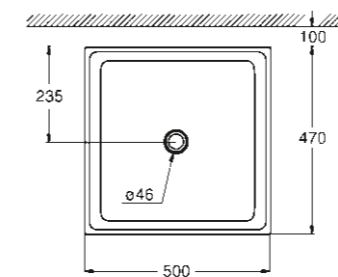
39 481 00H Vasque 50 cm
